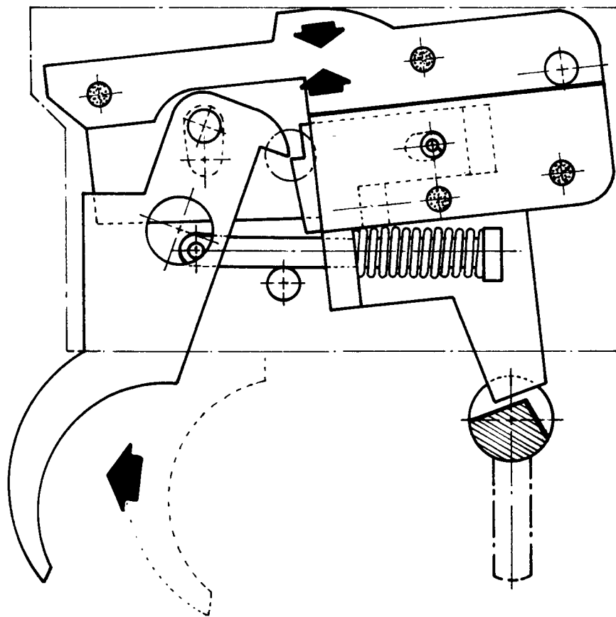
SEMI AUTO.
